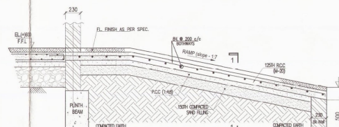
TYP. DET. OF RAMP
