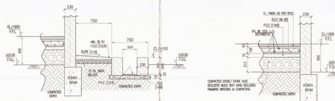
TYP. DET. OF FLOORING
