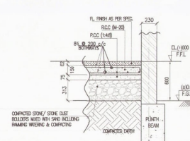
TYP. DET. OF FLOORING
